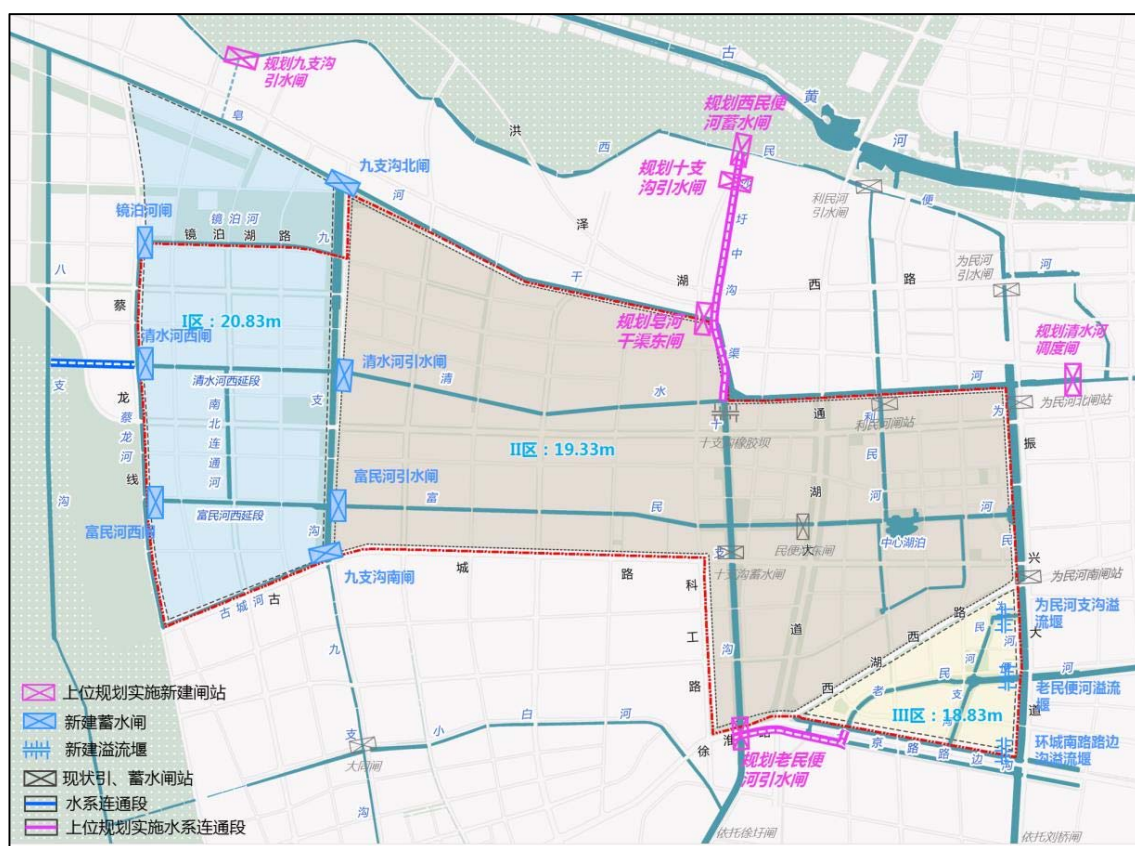
图 6.7-3 园区河道闸控规划建设布置图
